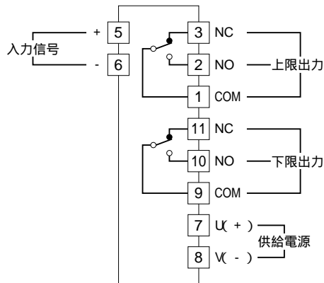
端子接続図
