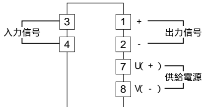
端子接続図
