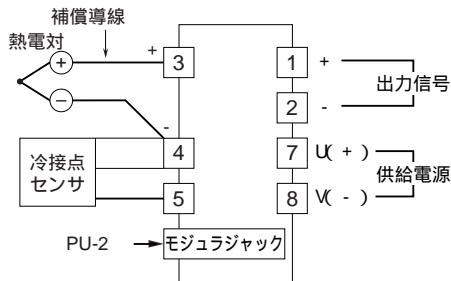
端子接続図
