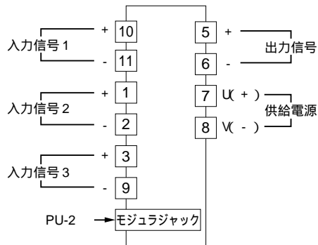
端子接続図
