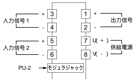
端子接続図
