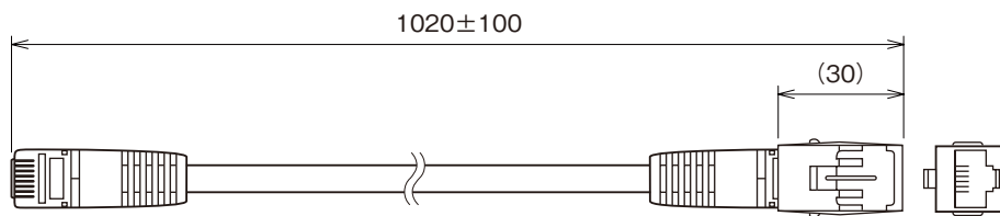
外形寸法図 (単位: mm)
