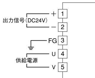
端子接続図
