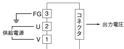
端子接続図
