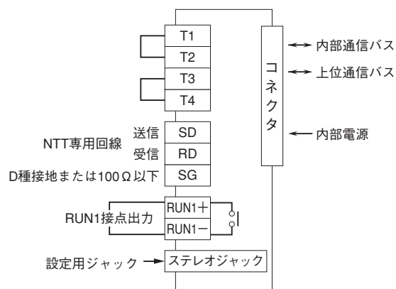
端子接続図
