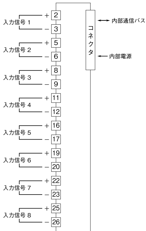
端子接続図
