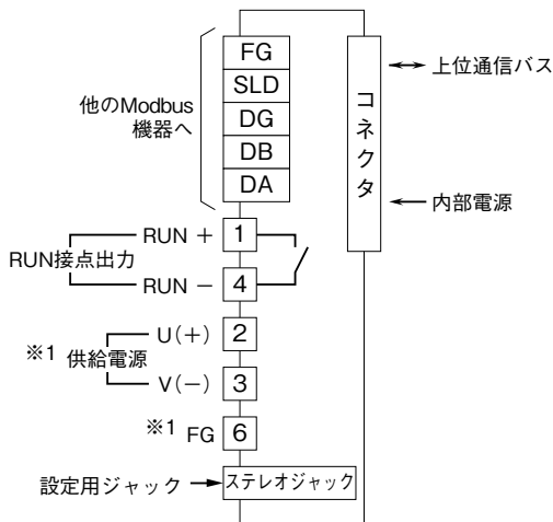
端子接続図
