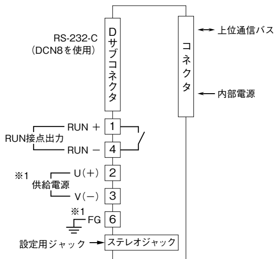
端子接続図
