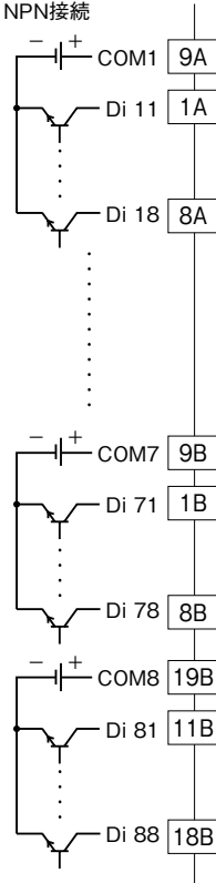
NPN接続
