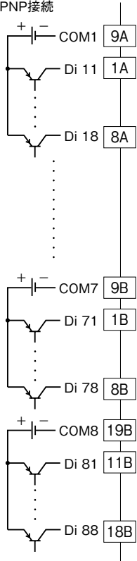
PNP接続
