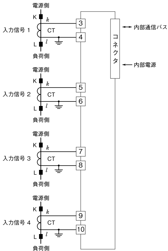
端子接続図
