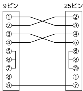
配線図
