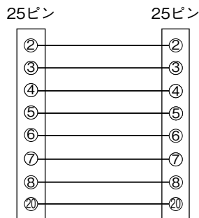
■配線図
