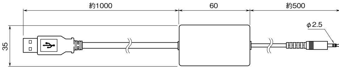
外形寸法図 (単位: mm)
