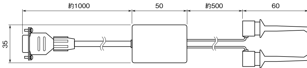
外形寸法図 (単位: mm)
