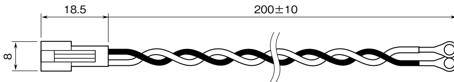
外形寸法図 (単位: mm)
