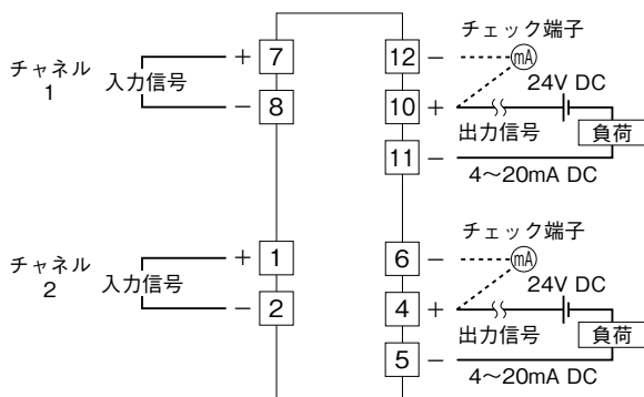
端子接続図
