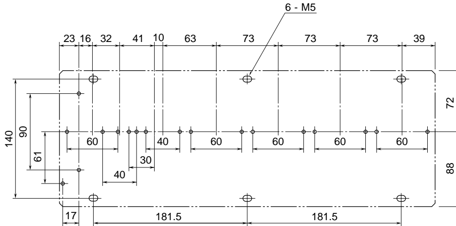
取付寸法図 (単位: mm)
