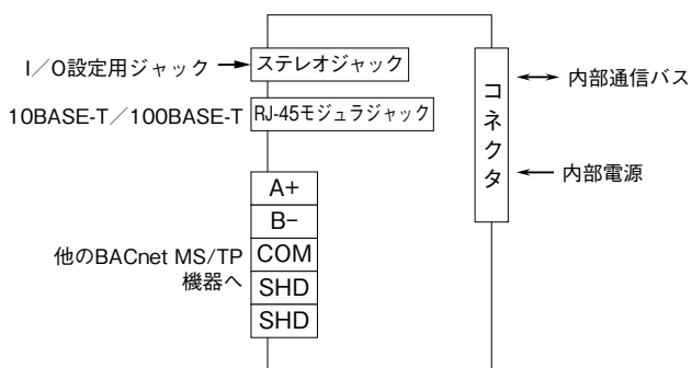
端子接続図
