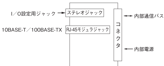
端子接続図
