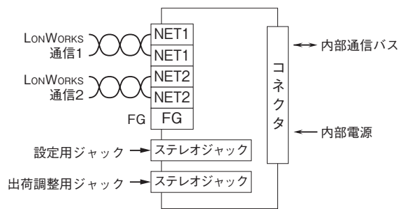
端子接続図
