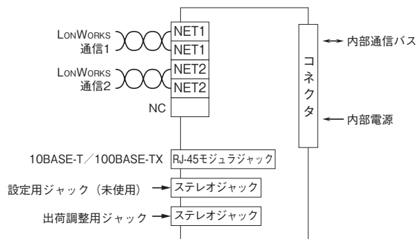
端子接続図
