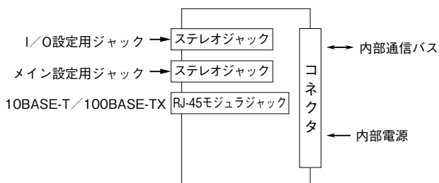
端子接続図
