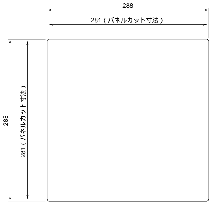
前面図
