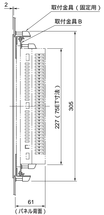
側面図
