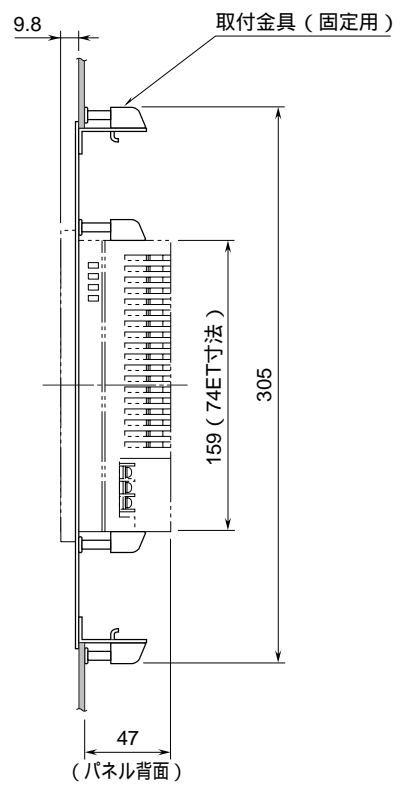
側面図
