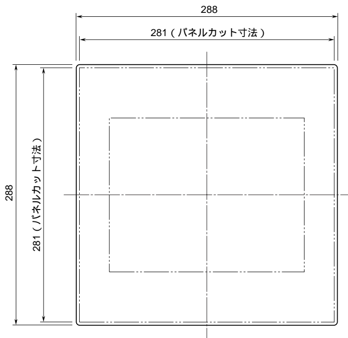
前面図
