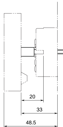
27・UNIT + 6DV 取付 (形式: A - 6 - 27)
