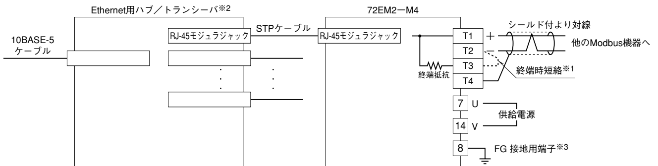
端子接続図
