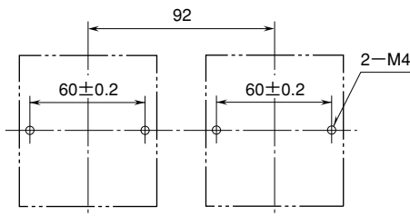
取付寸法図 (単位: mm)
