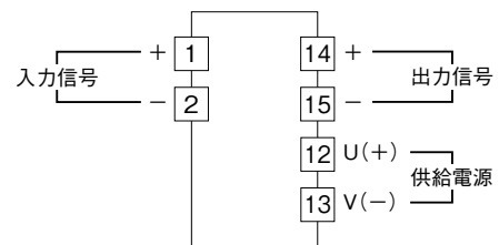
端子接続図
