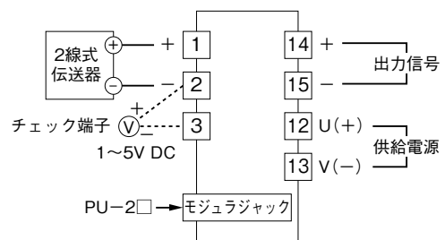
端子接続図
