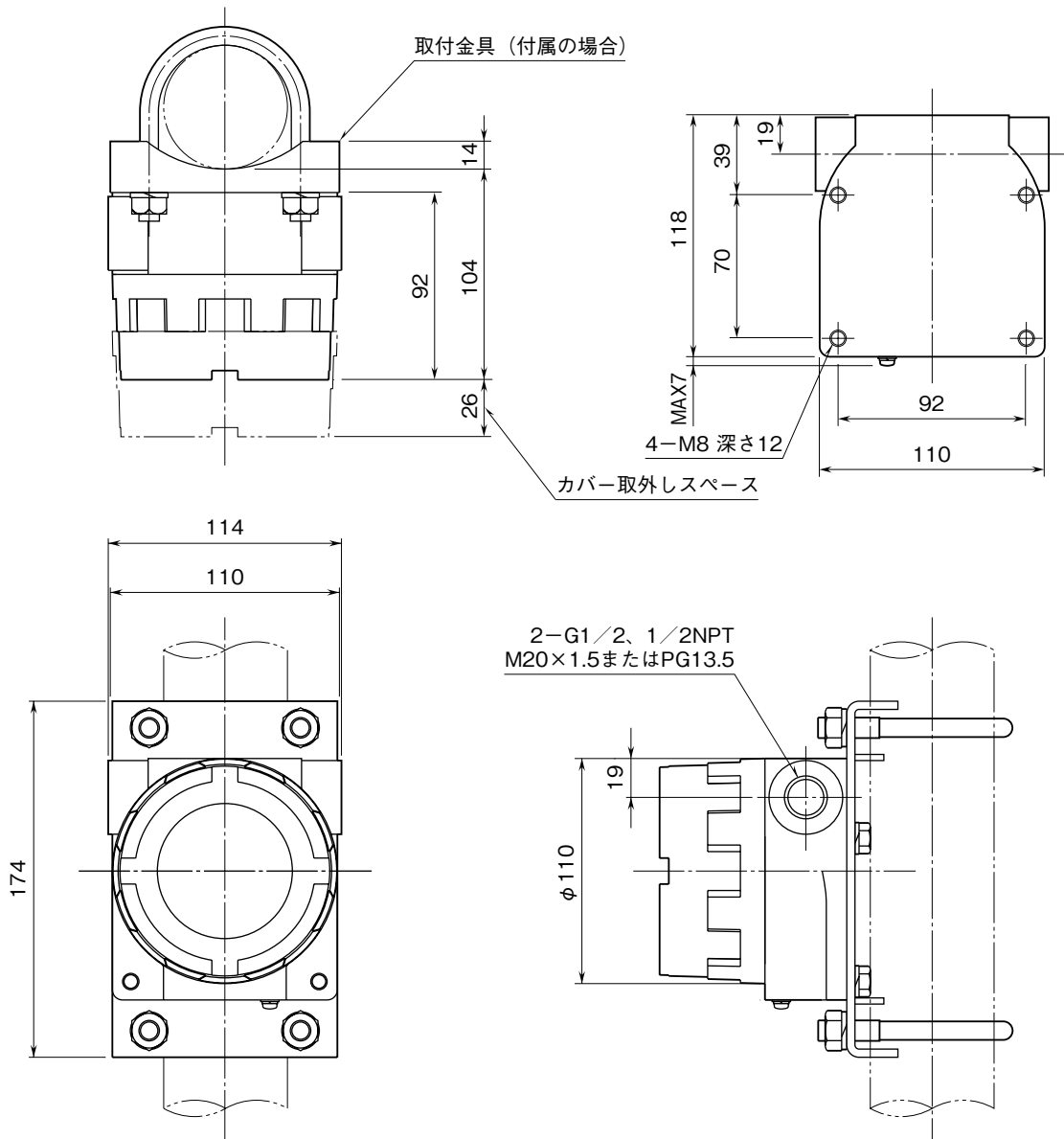
外形寸法図 (単位: mm)
