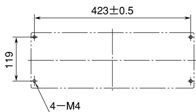
取付寸法図 (単位: mm)
