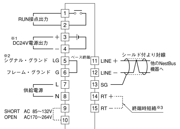
CPUモジュールのNestBus・電源端子接続図
