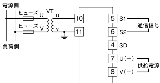
端子接続図
