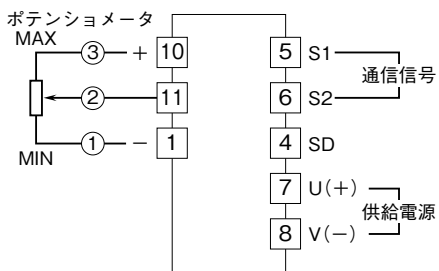
端子接続図
