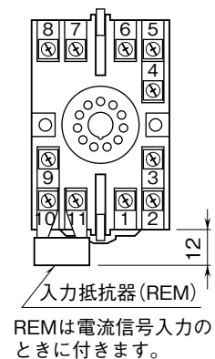
端子番号図 (単位: mm)
