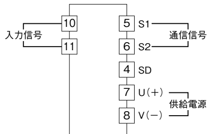
端子接続図
