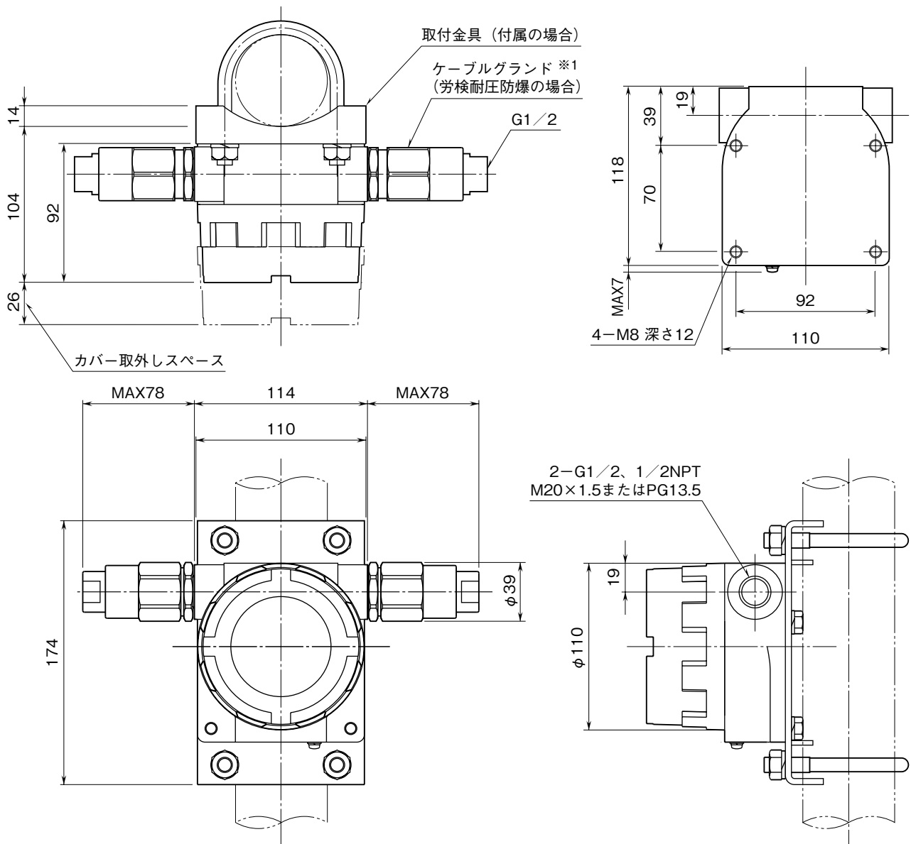
外形寸法図 (単位: mm)
