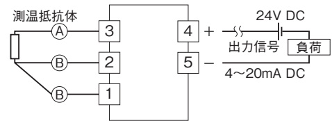
端子接続図
