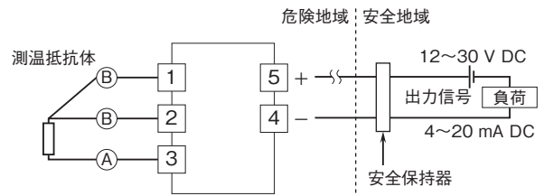
端子接続図
