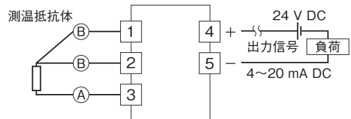
端子接続図
