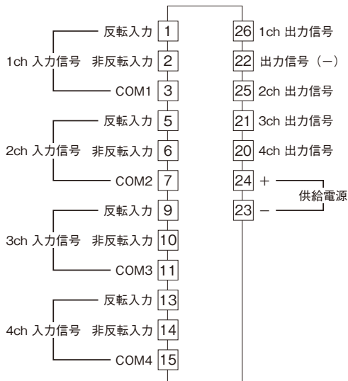
端子接続図
