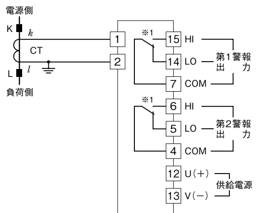
端子接続図
