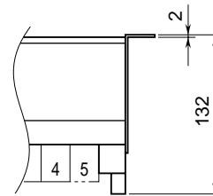
壁取付の場合 (付加コード: /W)
