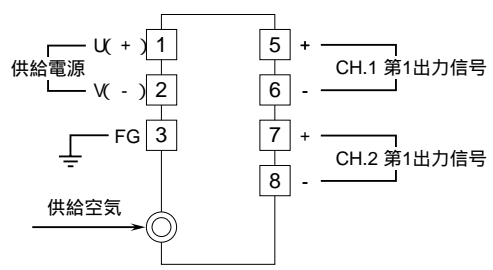
端子接続図
