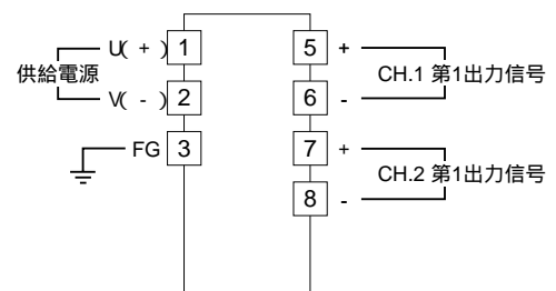
端子接続図
