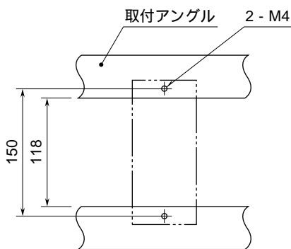
取付寸法図 (単位: mm)
