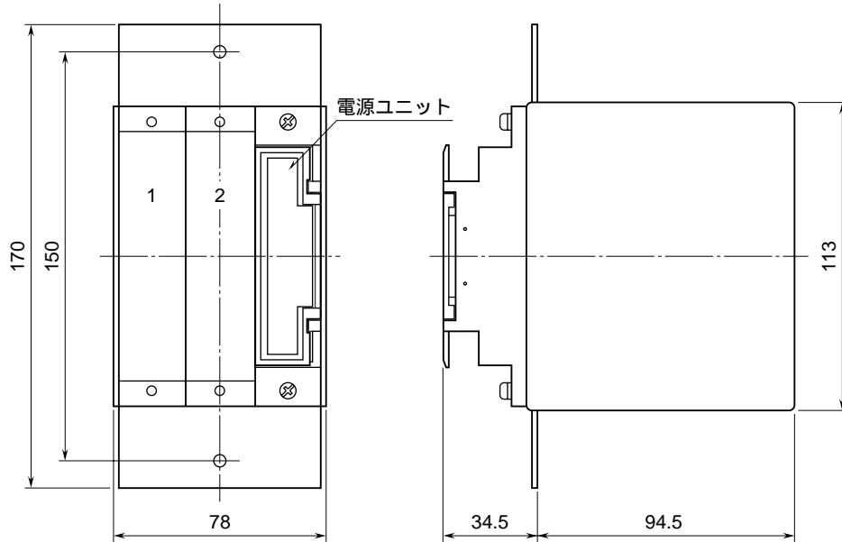
外形寸法図 (単位: mm)
