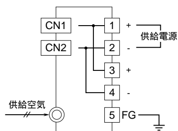
端子接続図
