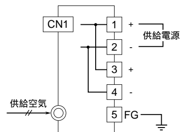
端子接続図
