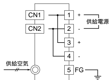
端子接続図
