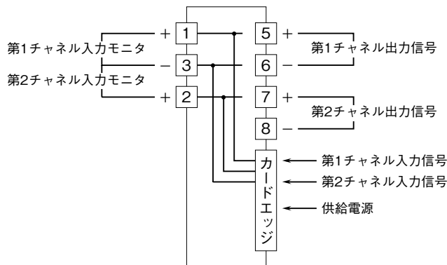
端子接続図
