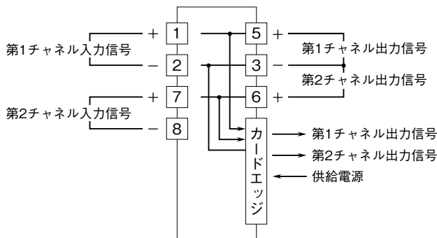
端子接続図
